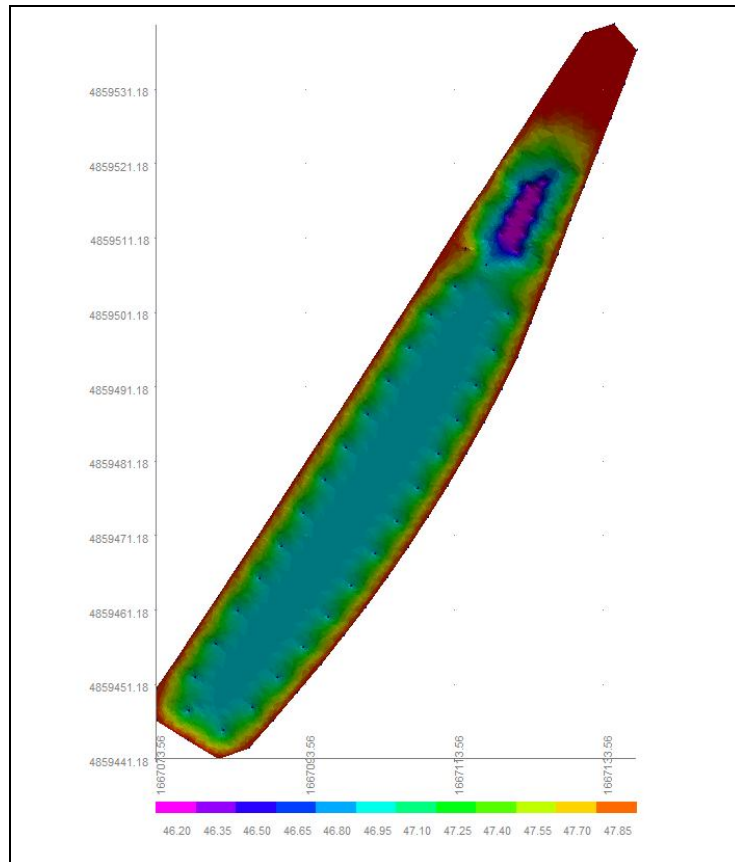
FIGURA 6 – MODELLAZIONE TRIDIMENSIONALE DELLA VASCA DI ACCUMULO
