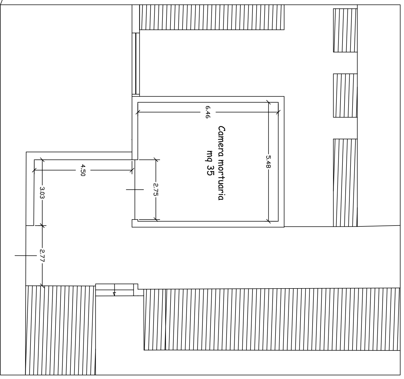
Planimetria locale presso Cimitero di Galciana Scala 1:100
